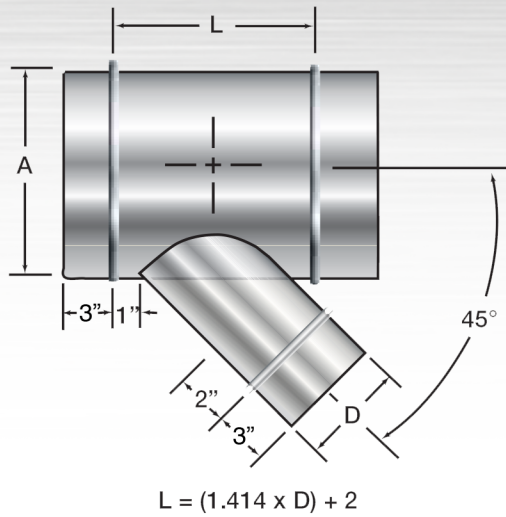
45° Lateral
